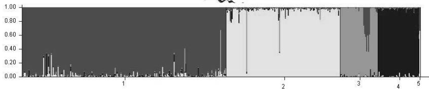
Obr. 2: Výstup z programu Structure pro čtyři klastery. Všechna čtyři plemena jsou dobře odlišena. Je zde viditelný také určitý genový tok mezi jednotlivými plemeny.
